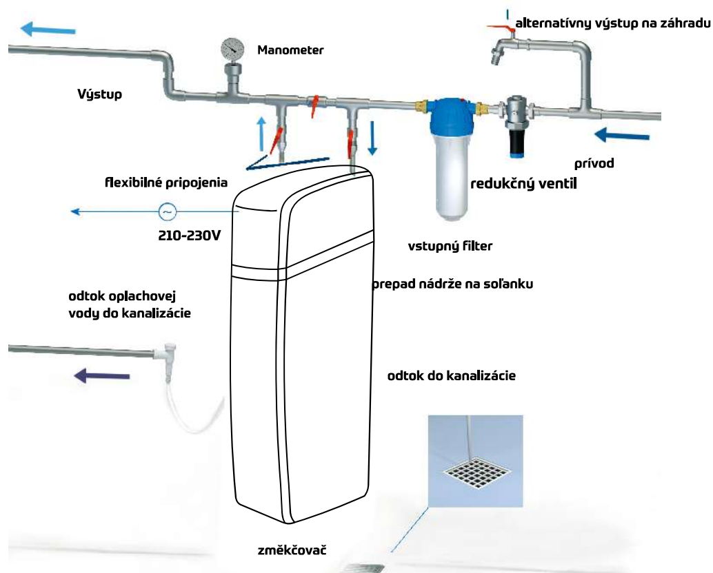
obr.2 Schéma zapojenia zmäkčovača
