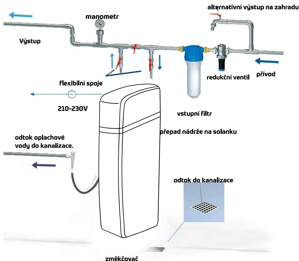
obr.2 Schéma zapojení změkčovače
